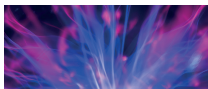
Plasmas
